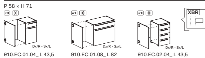
910.EC.01.04_ L 43,5 910.EC.01.08_ L 82 910.EC.02.04_ L 43,5
