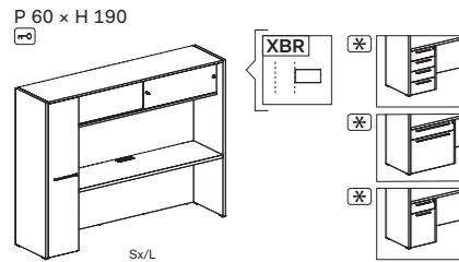
910.HC.01.25_ L 250 Dx/R - Sx/L
